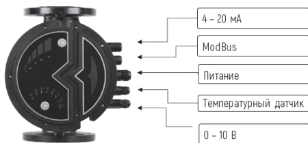
Рис. 7 Схема электроподключения насоса
