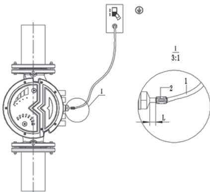
Рис. 6 Электроподключение
